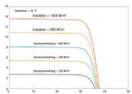
Strom-Spannungs-Kurve des Moduls M430N54LM-BF-F3
